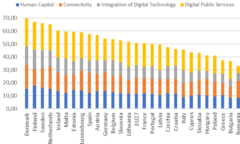
Figura 2 DESI 2021
